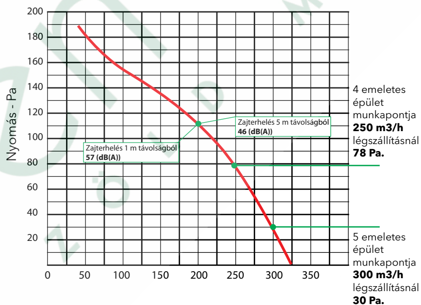
Ventilátor jelleggörbe
